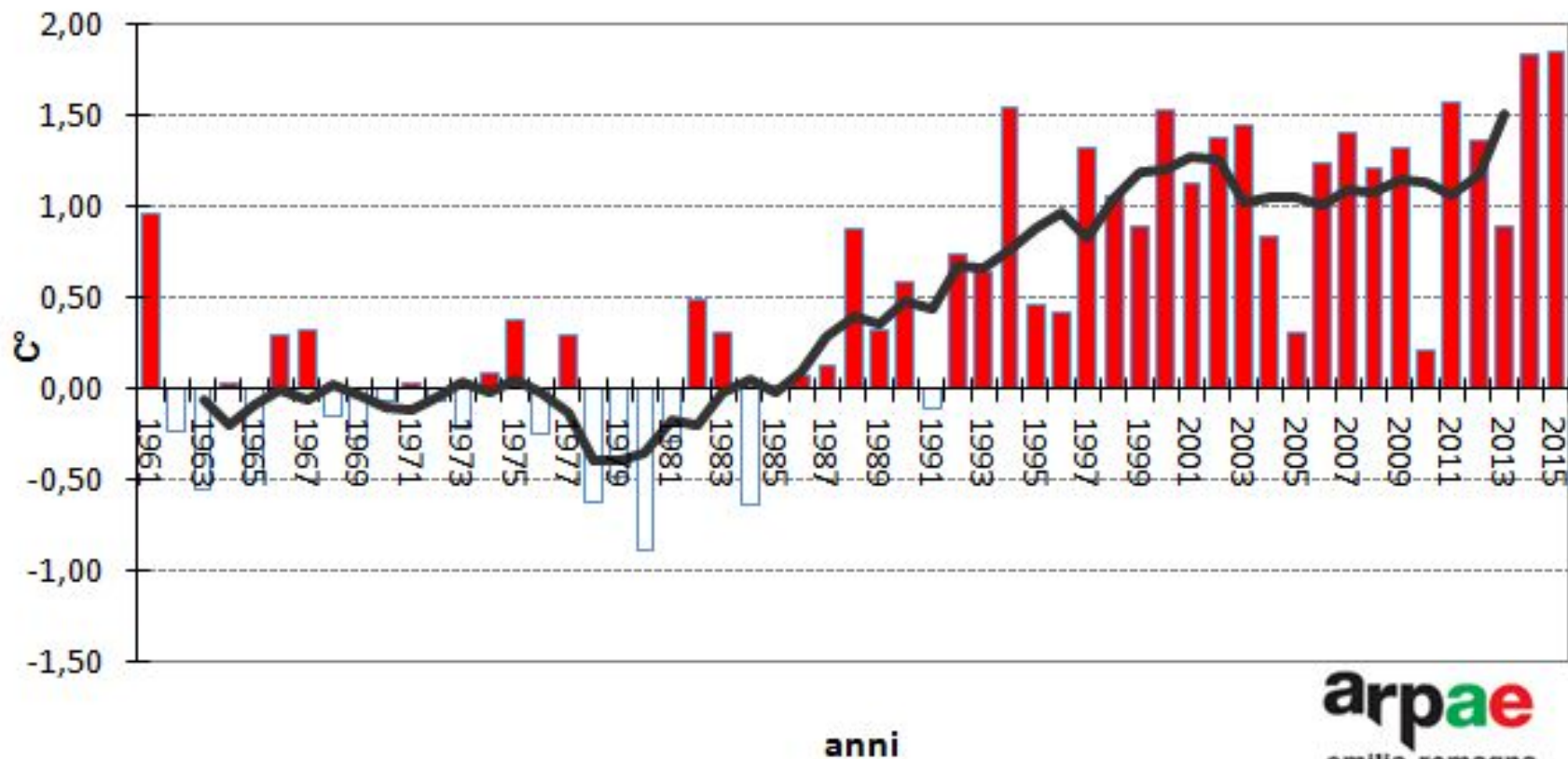
Scarto medio annuale della Tmed in Emilia-Romagna clima di riferimento 1961-1990
